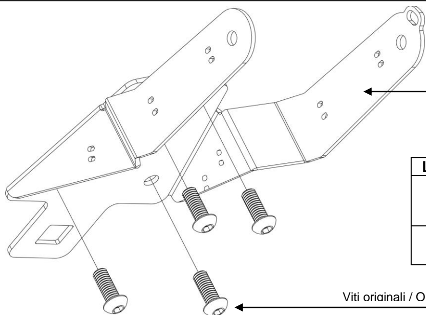
Piastra fissaggio portatarga / License Plate Support
